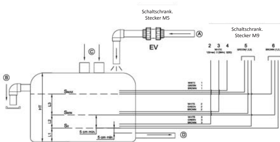
Installationsdiagramm für das Wasserschloss
