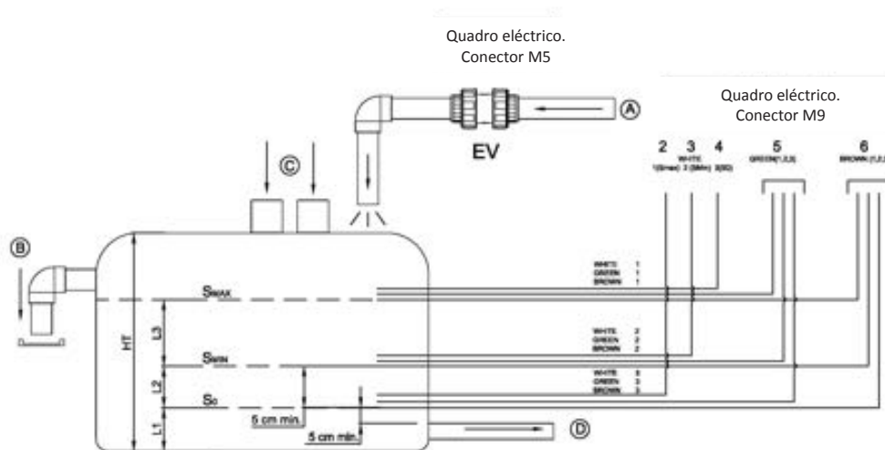
Diagrama de instalação do tanque de compensação.
