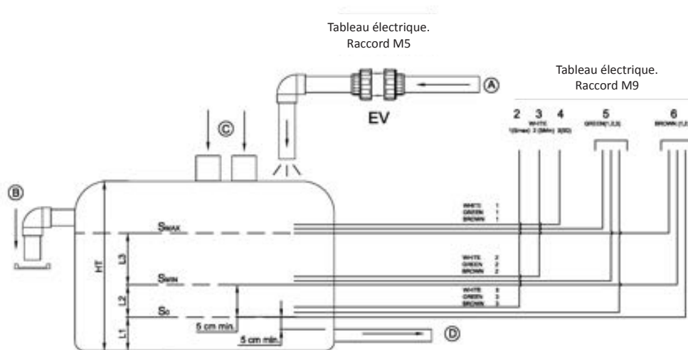
Schéma d'installation de la chambre d'équilibre.
