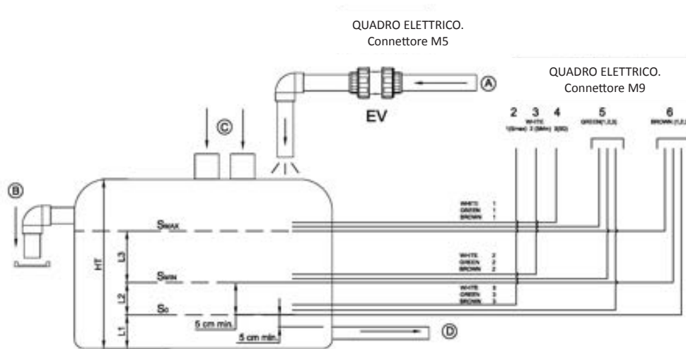
Schema installazione Vasca di compenso.
